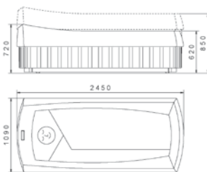
Thermo-Spa Designerverkleidung
